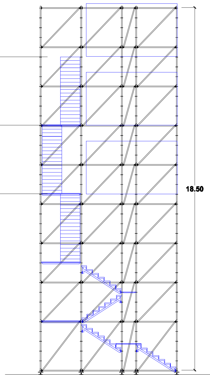
ALZADO LATERAL IZQUIERDO
