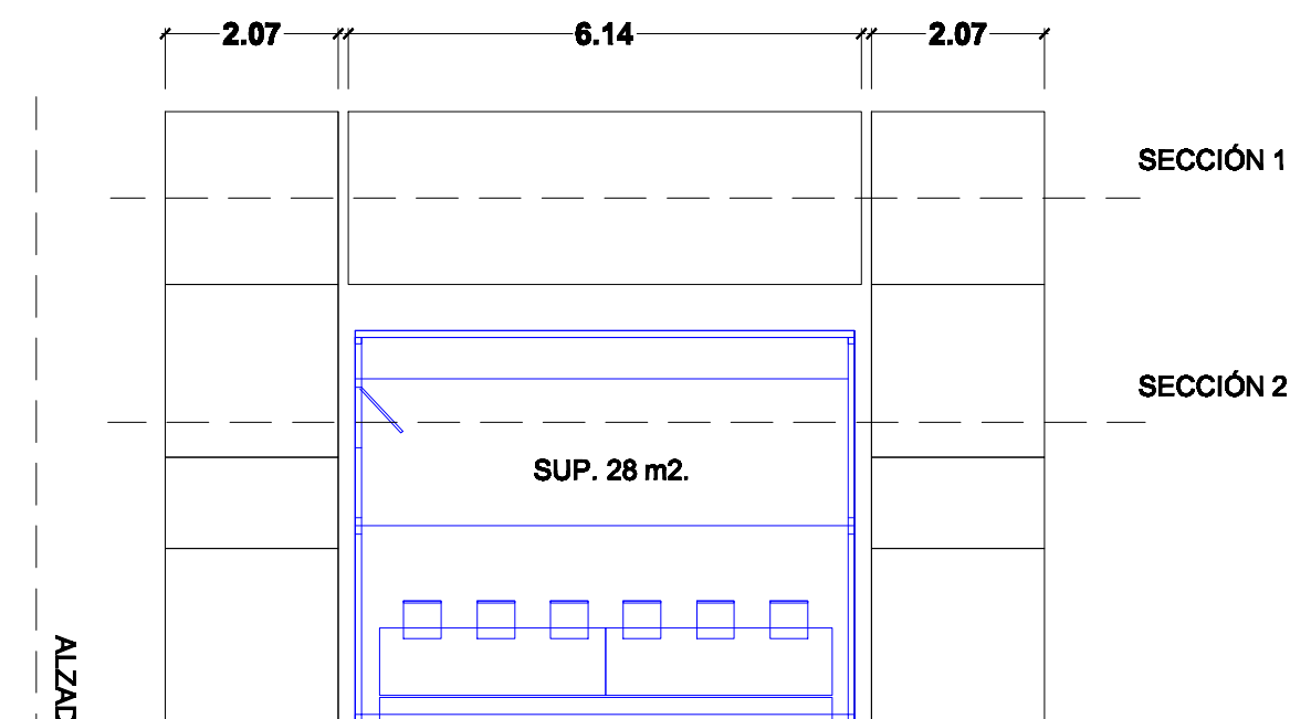
ALZADO
