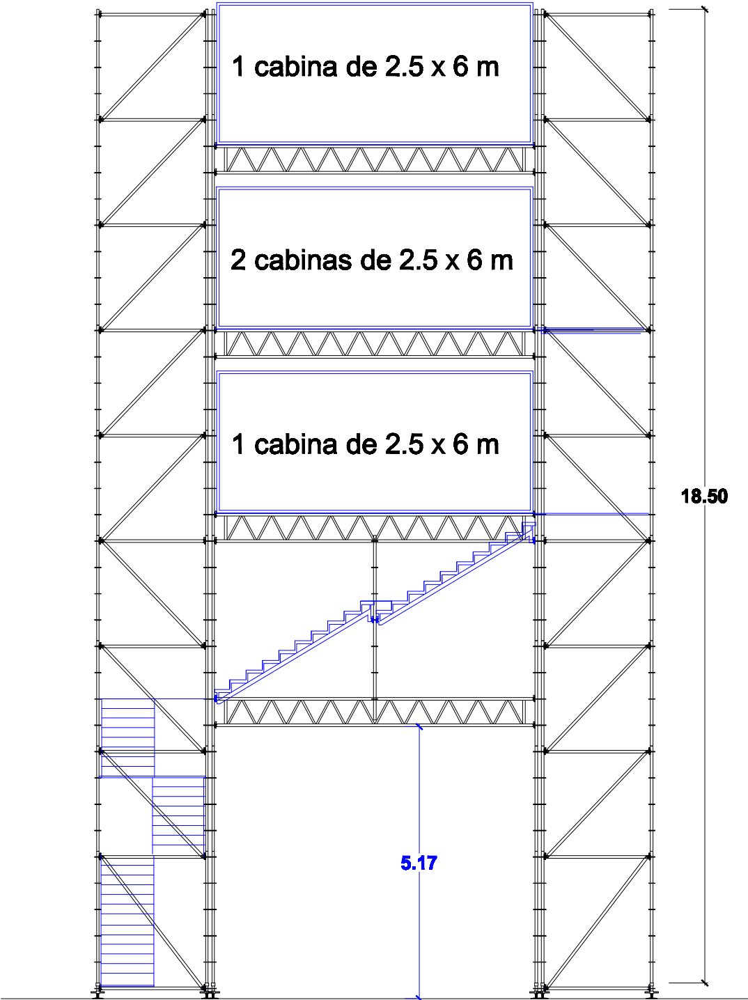
SECCIÓN 2
