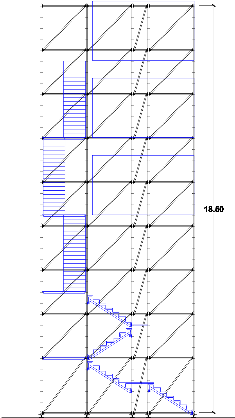
ALZADO LATERAL IZQUIERDO
