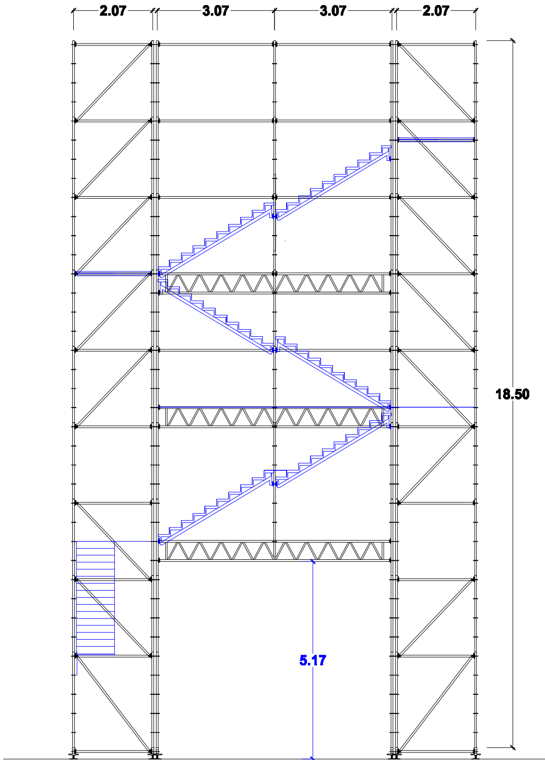
SECCIÓN 1
